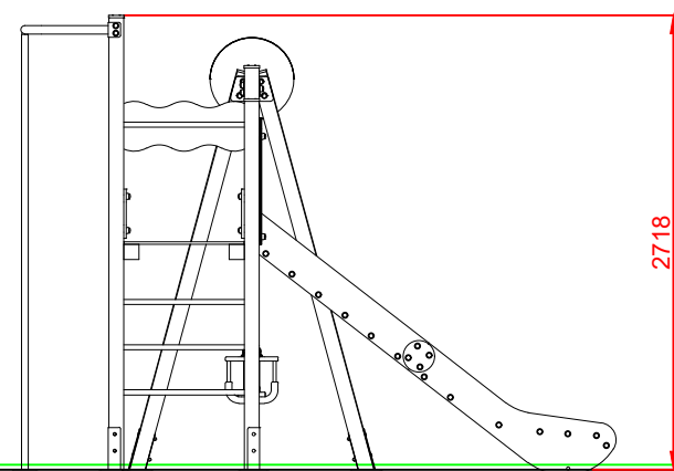
PERFIL IZQUIERDO
