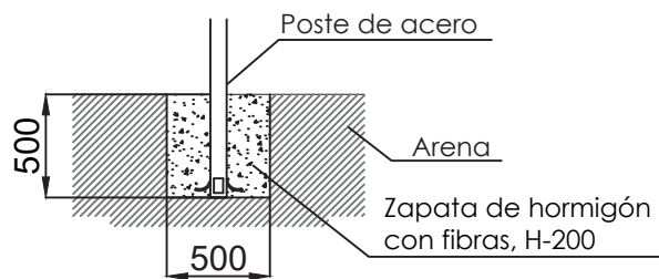
ESQUEMA DE CIMENTACIÓN POSTES
