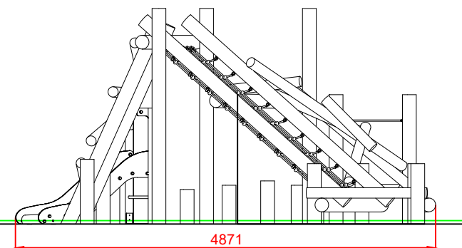
PERFIL
