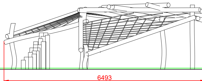
PERFIL
