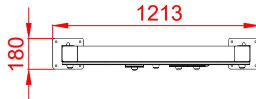
PLANTA
