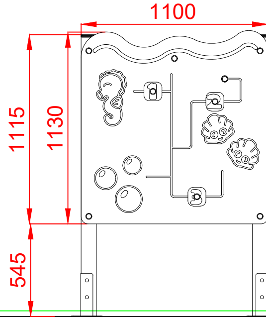
ALZADO
