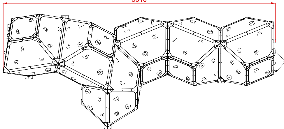
PLANTA
