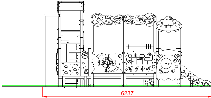
ALZADO
