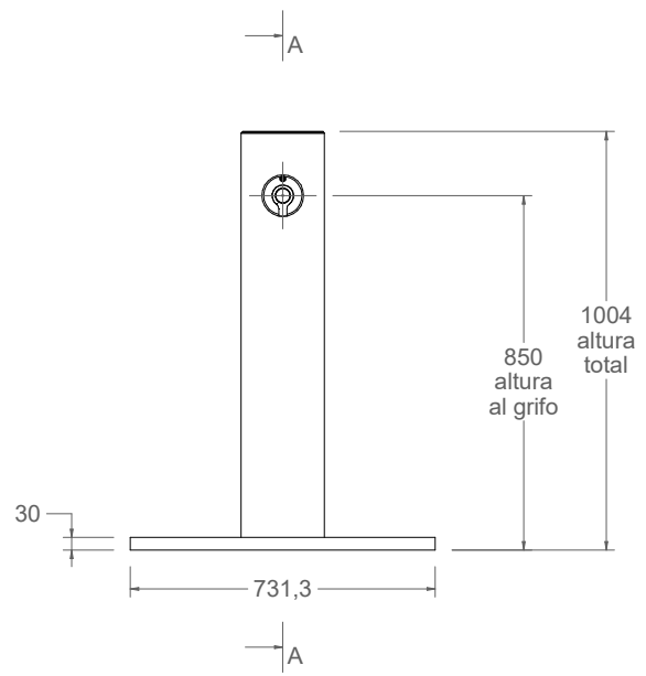
vista alzado 1:20
